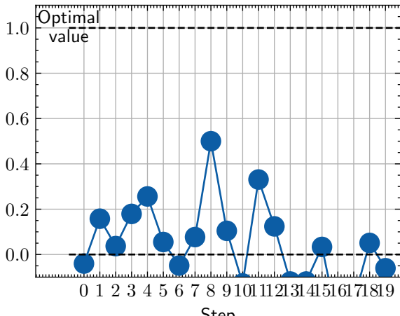
MulticlassCohenKappa
