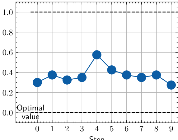
MultilabelRankingLoss
