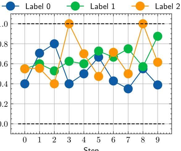
MultilabelPrecisionAtFixedRecall
