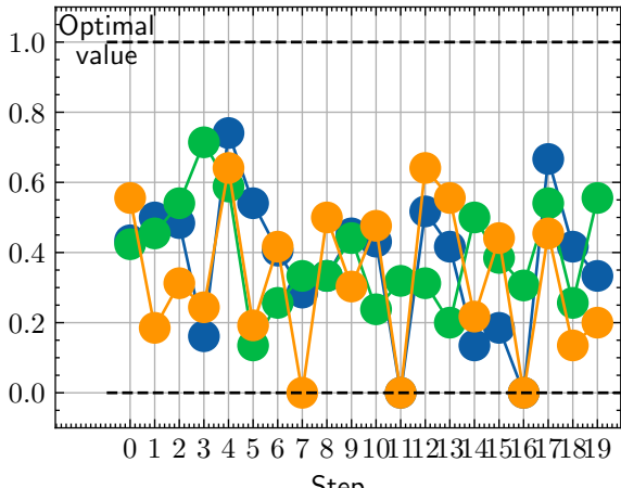
MulticlassFBetaScore
