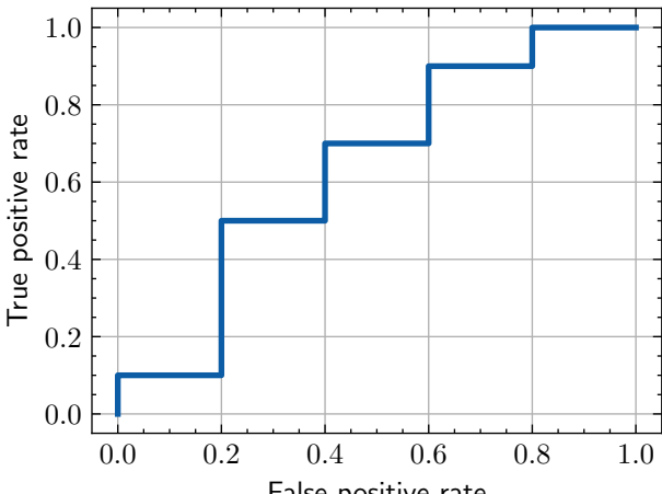
BinaryROC
