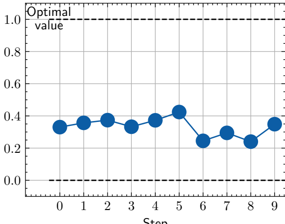
MultilabelJaccardIndex
