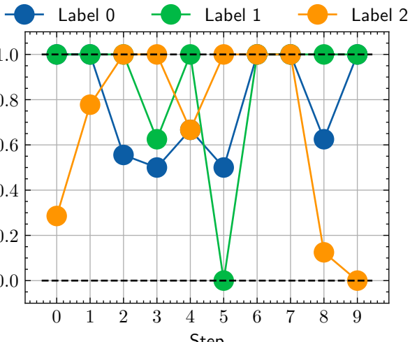
MultilabelRecallAtFixedPrecision
