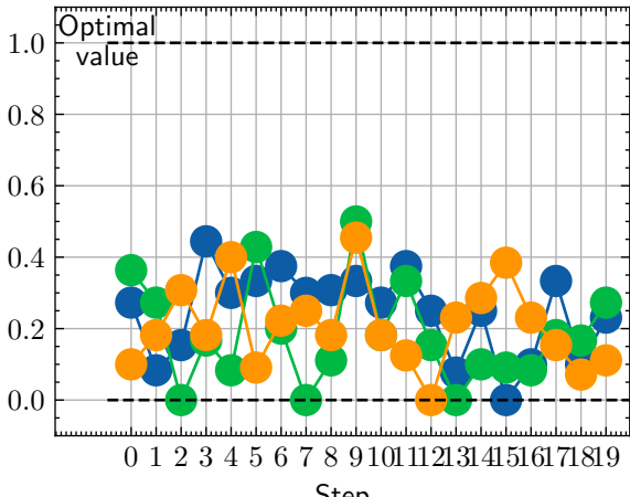
MulticlassJaccardIndex
