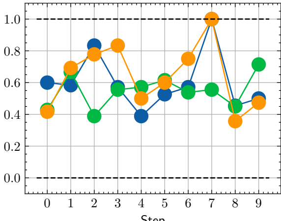
MultilabelPrecisionAtFixedRecall
