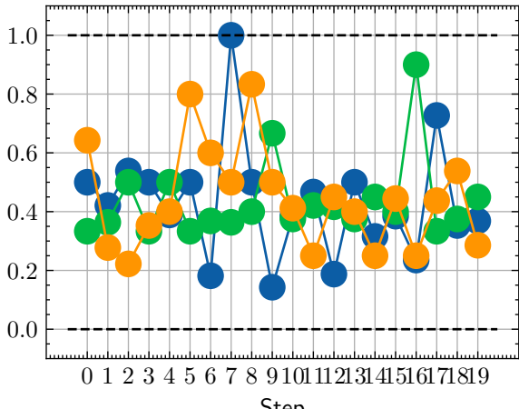
MulticlassPrecisionAtFixedRecall
