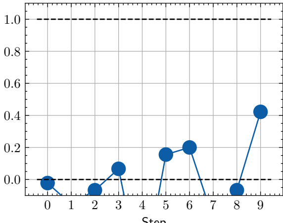
KendallRankCorrCoef
