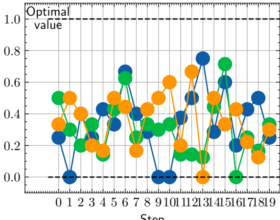
MulticlassPrecision
